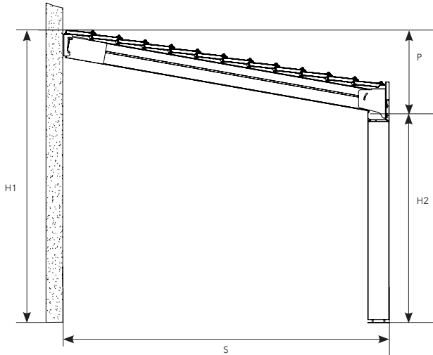
Yandan Görünüş / Side View
